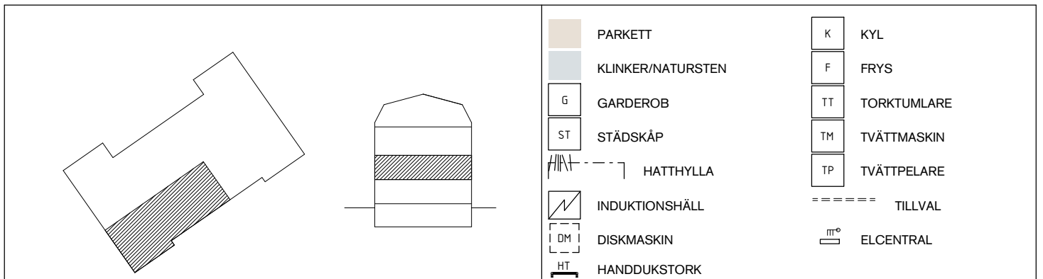
SKALA 1:100 (A4-FORMAT)
